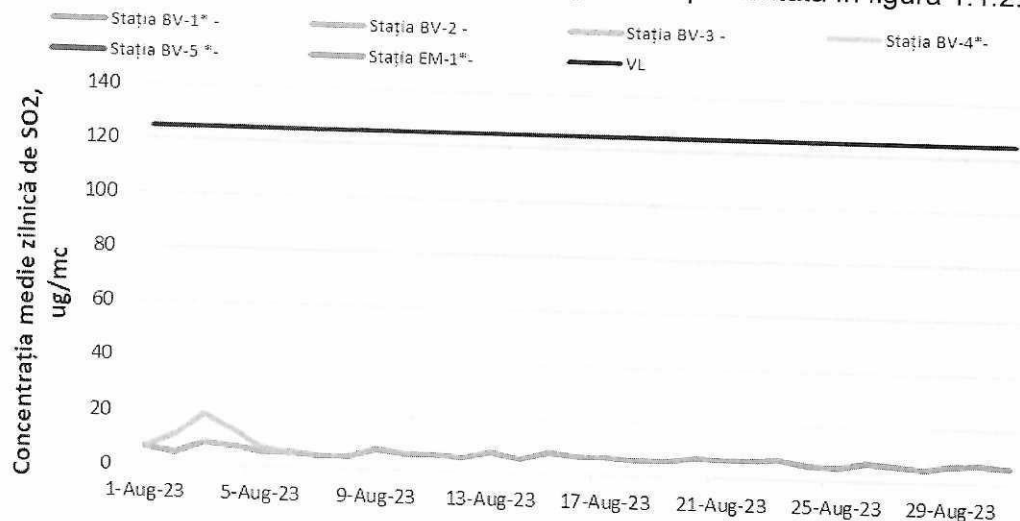
Figura 1.1.2.1.1. Evoluția mediilor zilnice de \text{SO}_2 în luna august
