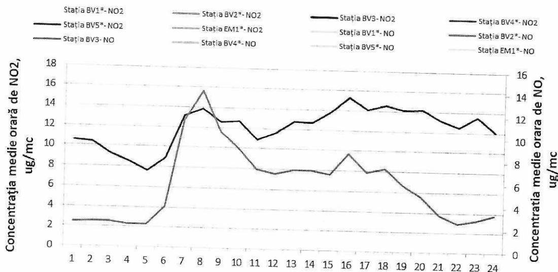
Figura 1.1.2.2.2. Ciclul zilnic al NO 2 și NO
