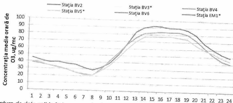
*captura de date valide în luna august a fost de 0% la stația BV3, la stația BV5 și la stația EM1 din motive tehnice Figura 1.1.2.3.3. Ciclul zilnic al ozonului
